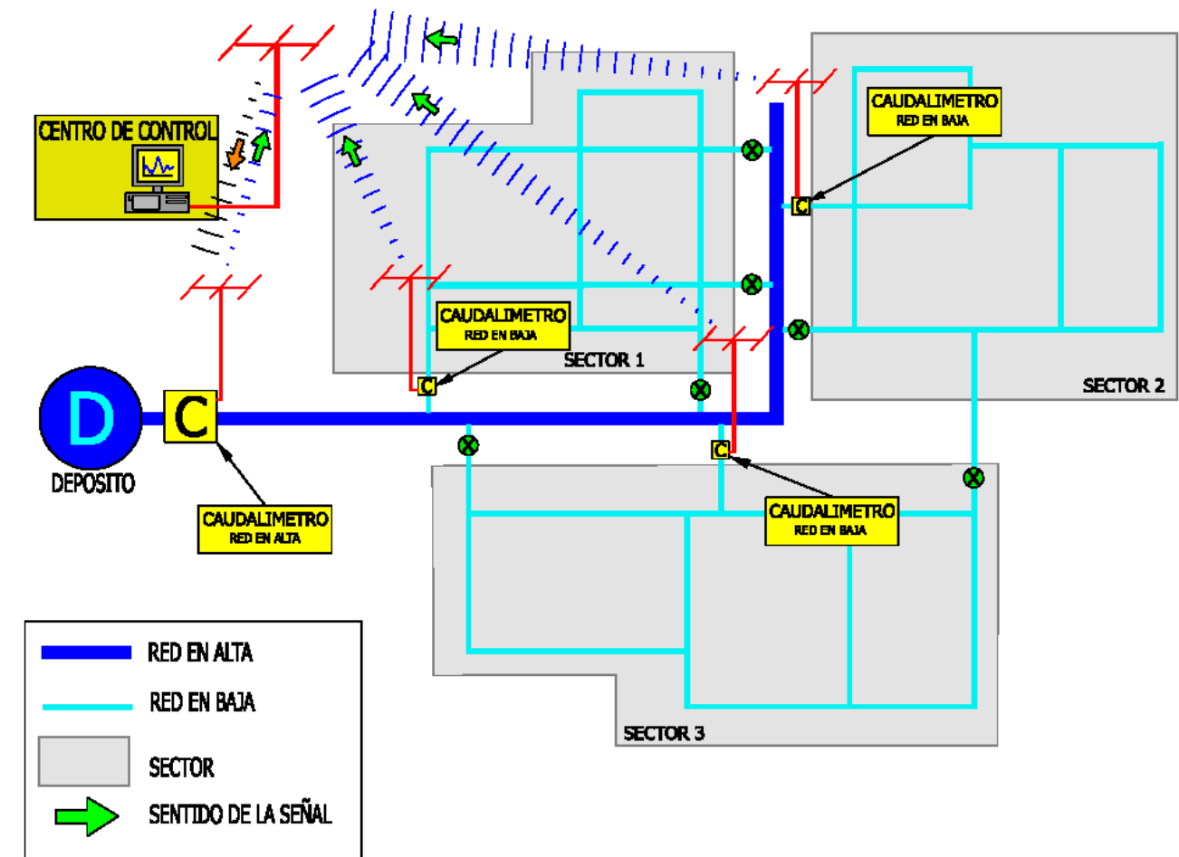
ESQUEMA DEL SISTEMA DE SECTORIZACION
