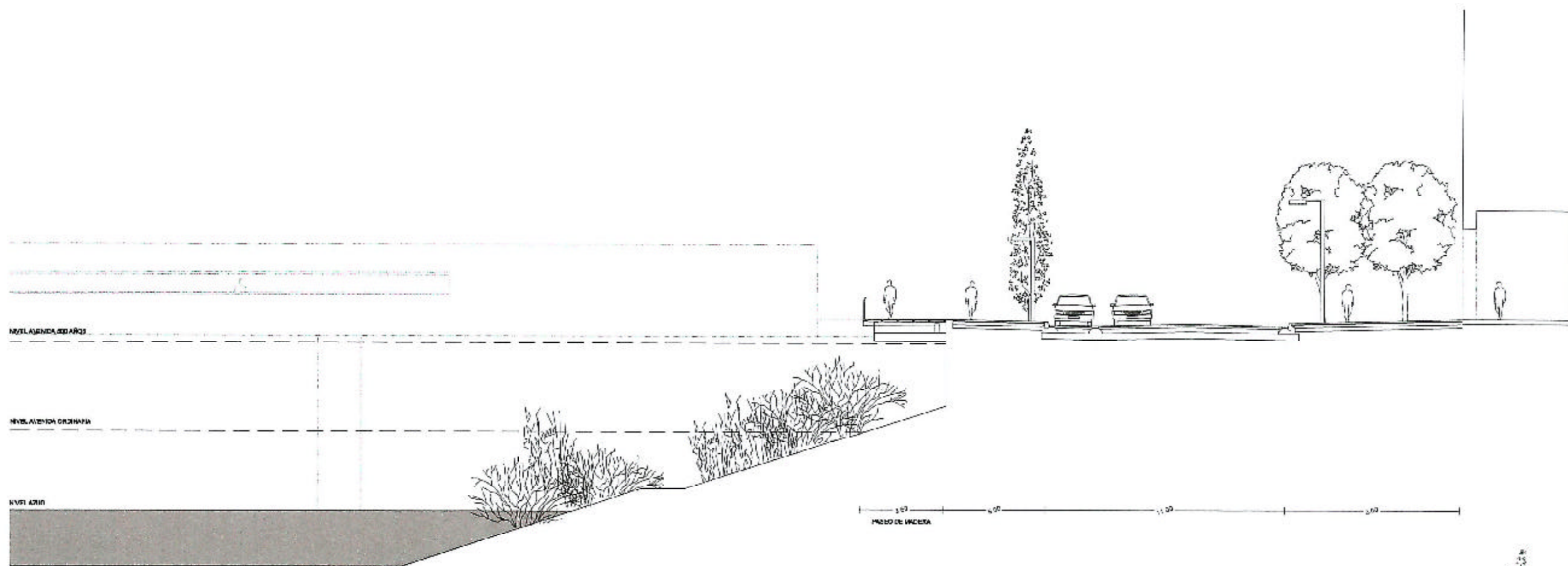
SECCION TIPO PASEO DEL EBRO (RIBERA IZQUIERDA) TRAMO PASEO ECHEGARAY Y CABALLERO
