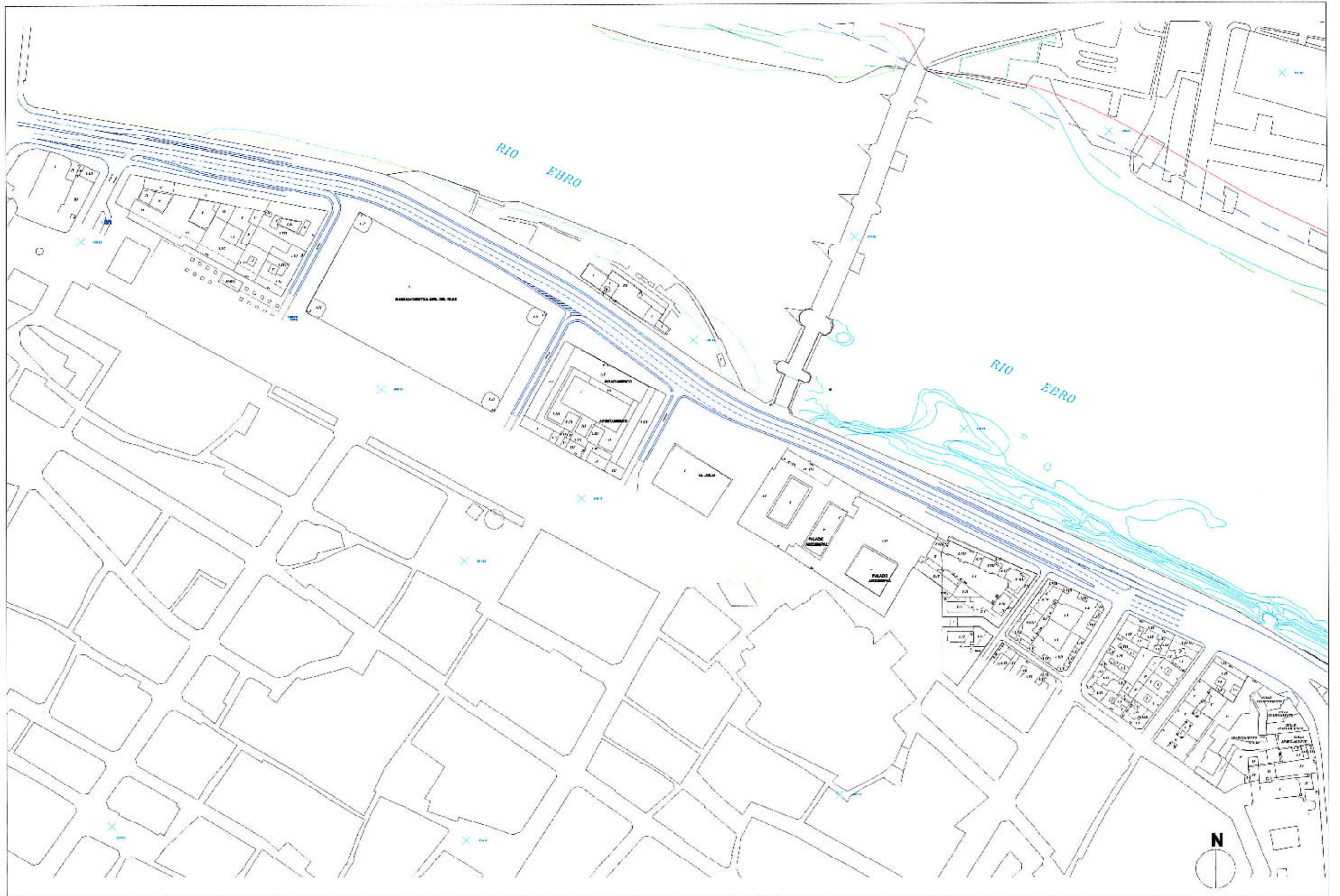
Balcón del Pilar-Echegaray y Caballero. Planta túnel ESCALA 1/2.000 AVANCE DE ORDENACION PROYECTO RIBERAS DEL EBRO
